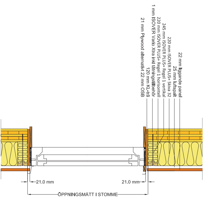
Vertikalsnitt, fönsterfästning KL-trä
